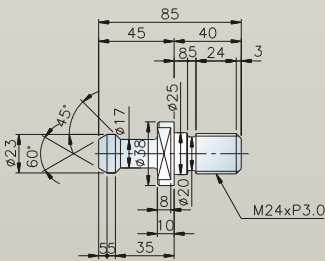
BT-50拉刀螺栓規格
