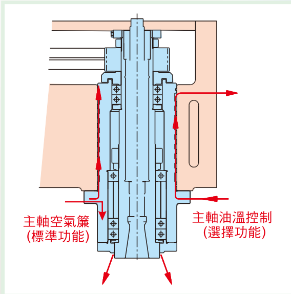
BT-40主軸
