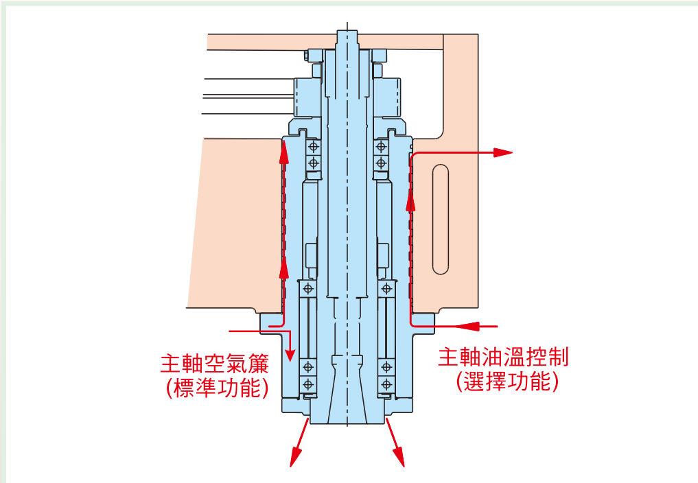
BT-40主軸
