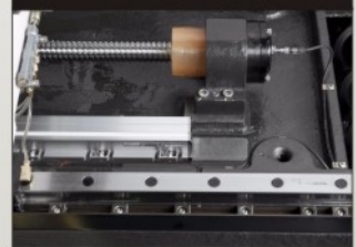
三軸光學尺
